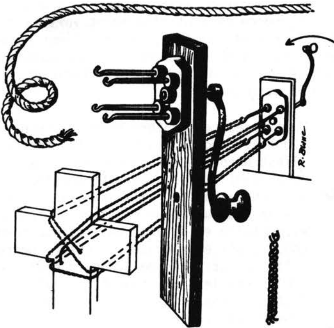
Le moulin à corder : c'est encore un appareil mais qui, par son mécanisme, annonce déjà la machine.
