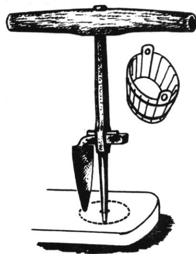
Un outil de boisselier: le couteau à rondelles
